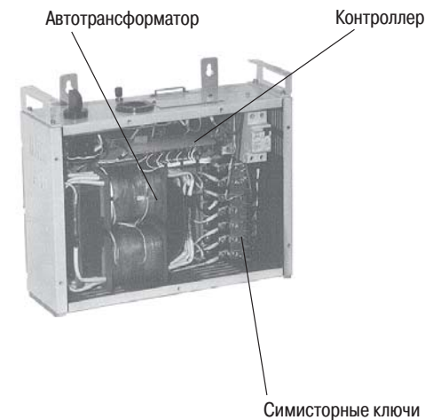
Рис. 8. Устройство стабилизатора
