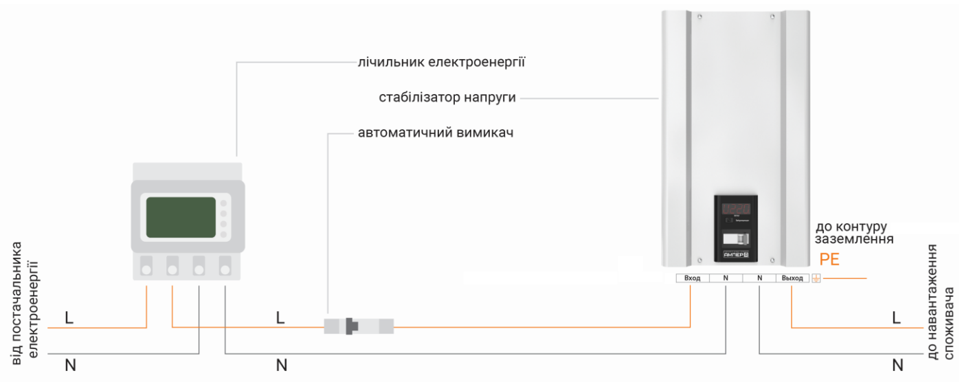
Рисунок 6. Схема підключення стабілізатора 25-80А до однофазної мережі
