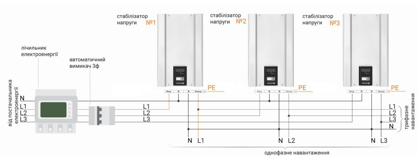
Рисунок 7. Схема підключення стабілізатора 25-80А до трифазної мережі
