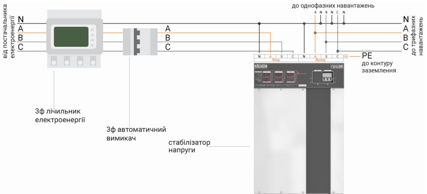
Рисунок 10. Схема підключення стабілізатора до трифазної мережі
