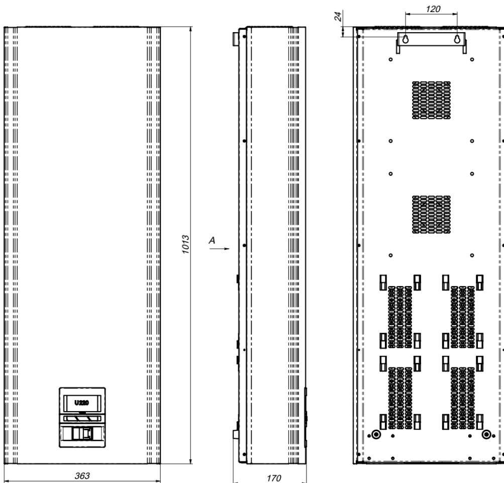
Рисунок 9. Установчі та посадочні розміри стабілізаторів Герц на 100-125А
