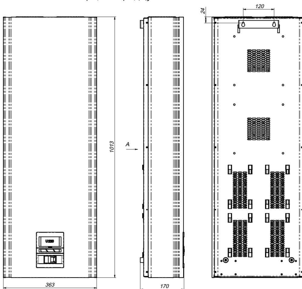
Рисунок 8. Установочные и посадочные размеры стабилизаторов Герц и Герц-Дуо на 50-63-80 А
