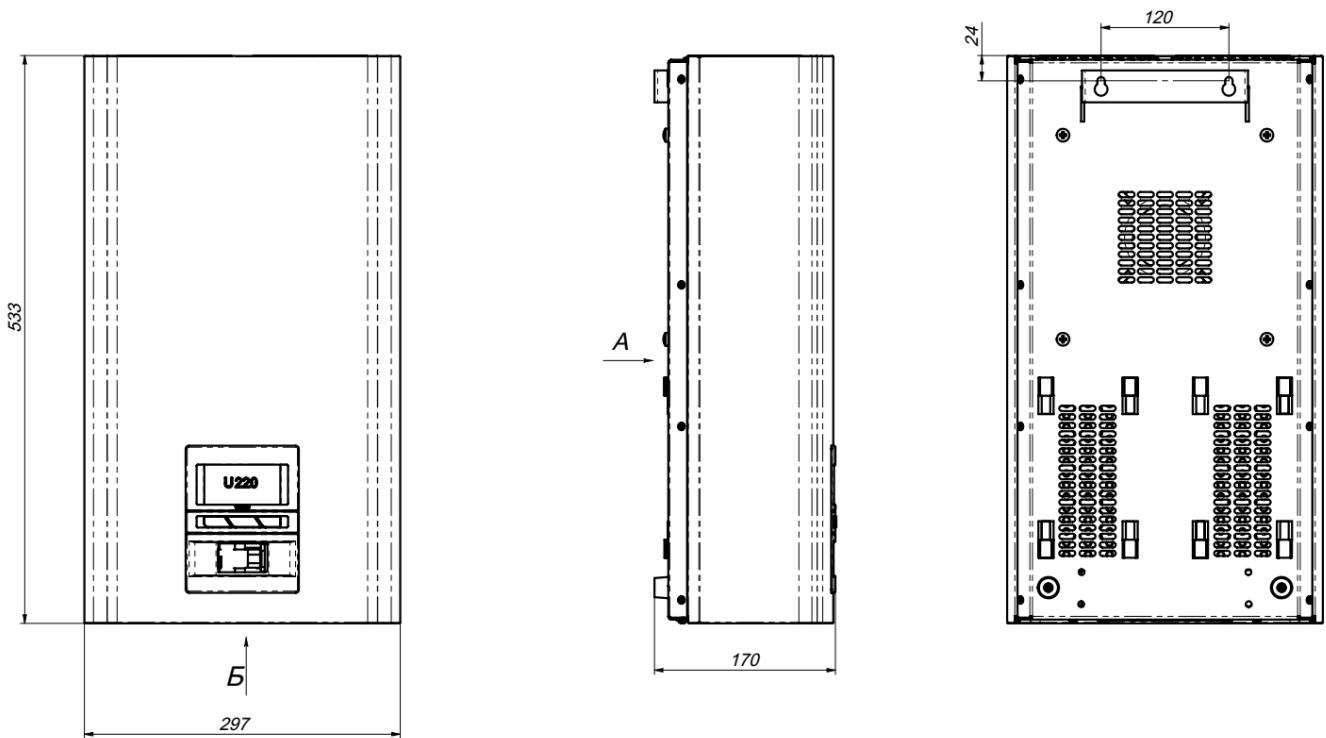
Рисунок 8. Установчі та посадочні розміри стабілізаторів
