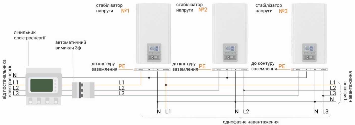
Рисунок 11. Схема підключення стабілізатора до трифазної мережі
