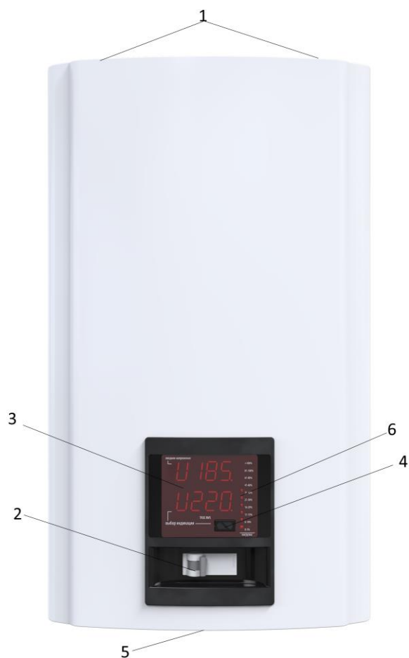
Рис.3 Зовнішній вигляд стабілізатора Герц-Дуо У 16-1/XXX V3.0
