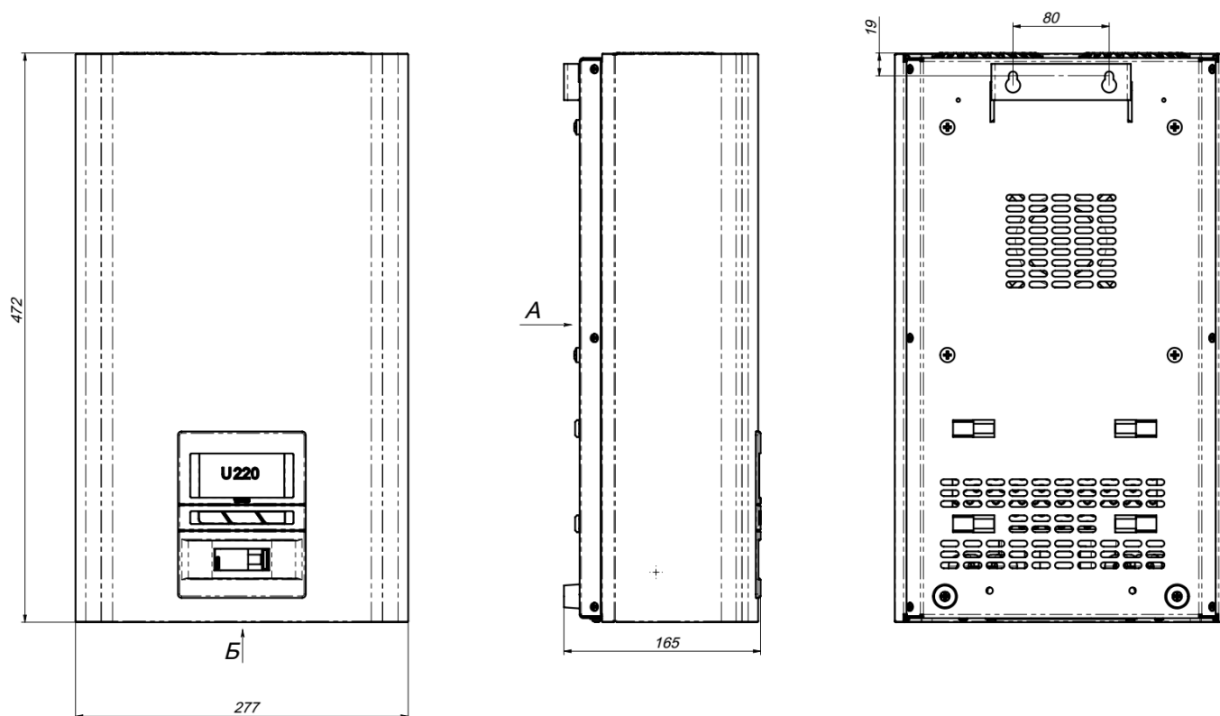
Рисунок 7. Установчі та посадочні розміри стабілізаторів Герц і Герц-Дуо на 25-32-40 А
