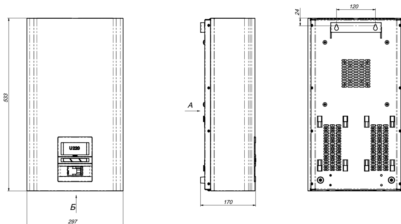
Рисунок 8. Установочные и посадочные размеры стабилизаторов Герц и Герц-Дуо на 50-63-80 А
