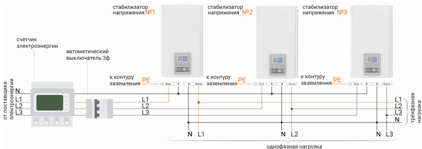
Рисунок 11. Схема подключения Герц и Герц-Дуо к трёхфазной сети
