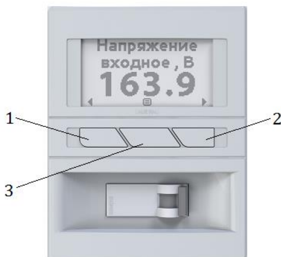
Рисунок 13. Расположение кнопок управления на панели управления Герц V3.0
