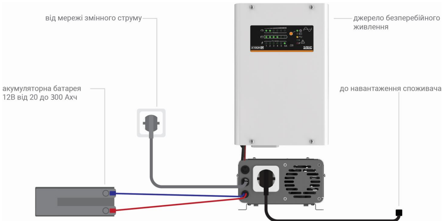
Рисунок 6. Схема підключення ДБЖ до силової мережі
