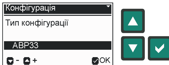
Рис. 5.19 – Меню «Конфігурація»
