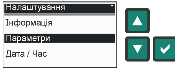
Рис. 5.14 – Меню «Налаштування»
