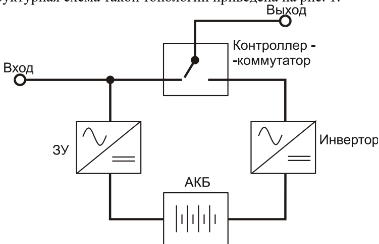
Рисунок 1. Структурная схема ИБП
