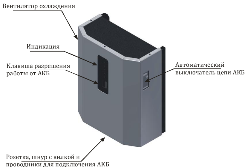
Рисунок 2. Внешний вид ИБП RESERVE–500 S
