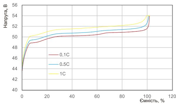
Криві заряду при різних струмах заряду (при 25°C)
