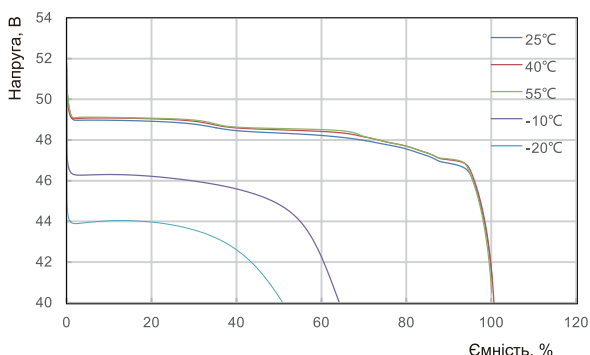
Криві розряду при різних температурах
