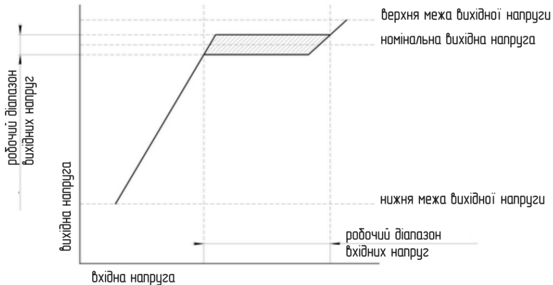
Малюнок 1. Передатна характеристика стабілізатора напруги.
