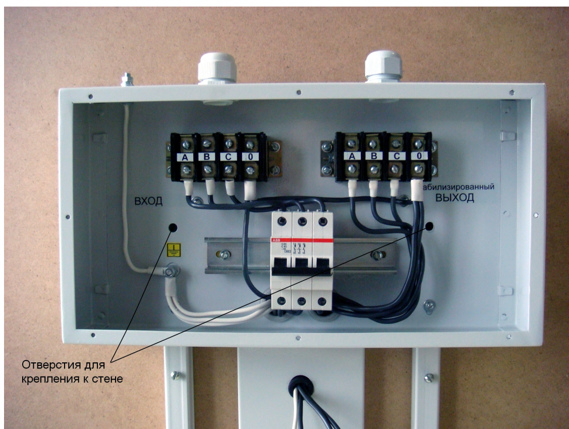
Рис.3. Коммутационный щиток.
