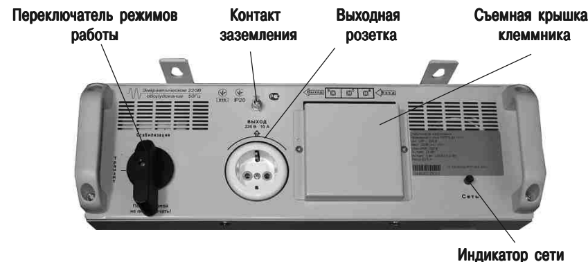
Рис. 4. Верхняя панель стабилизатора
